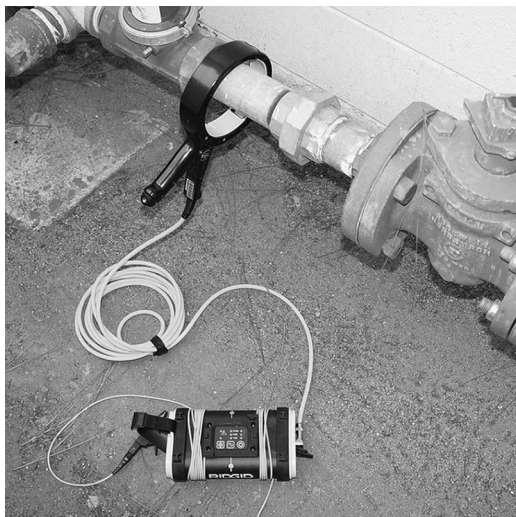
Рис. 9: Индукционный зажим присоединен к проводнику
